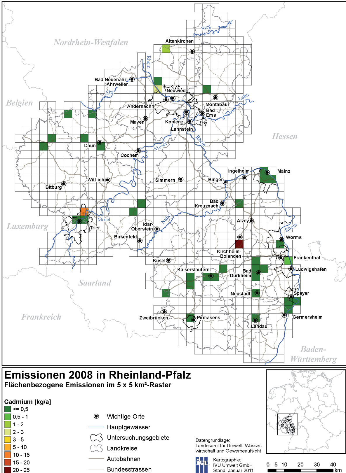
Abb. 58: Flächenbezogene Cadmium-Emissionen 2008 im 5 x 5 km 2 -Raster
