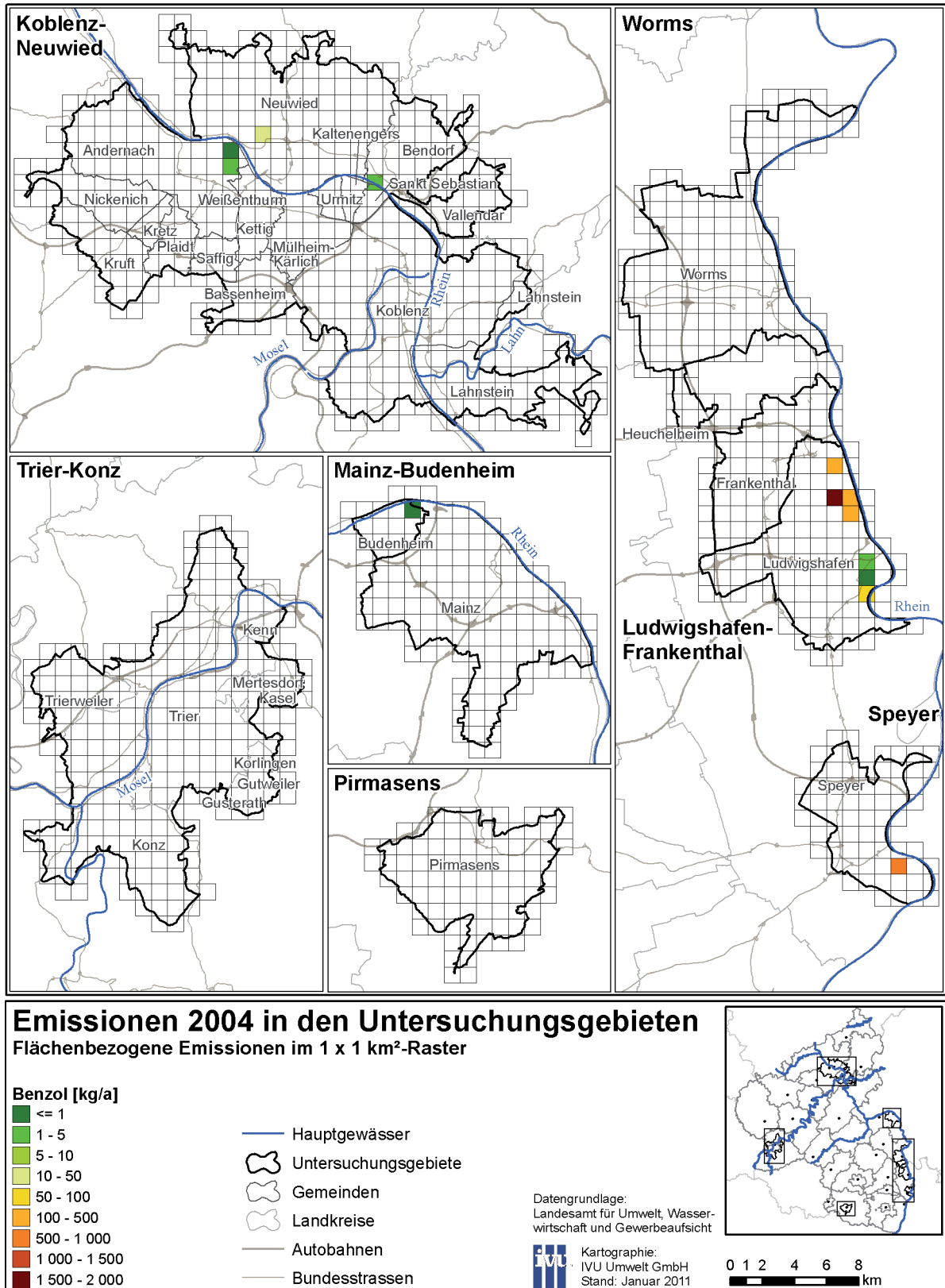
Abb. 73: Flächenbezogene Benzol-Emissionen in den Untersuchungsgebieten 2004 im 1 x 1 km 2 -Raster
