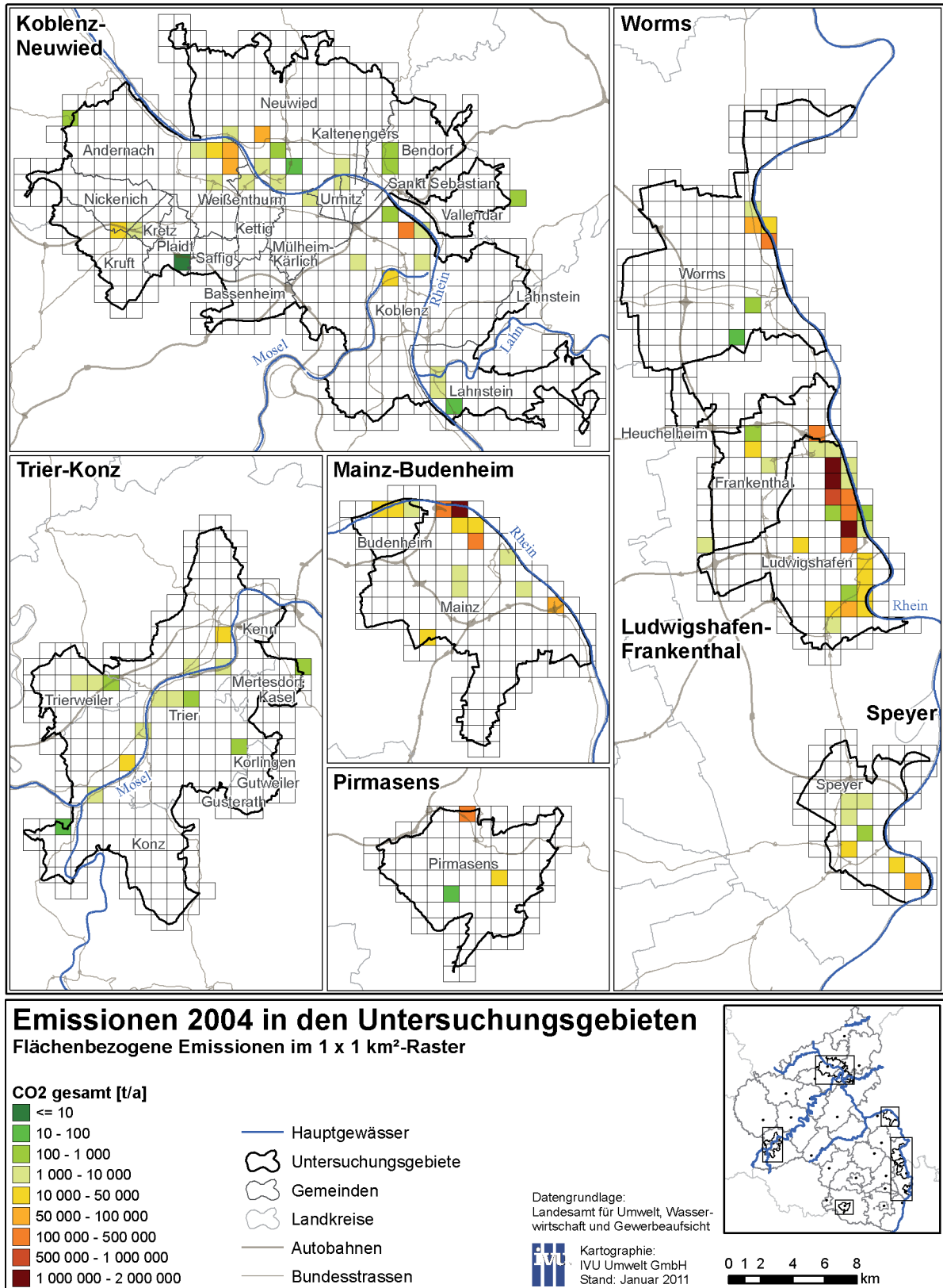
Abb. 61: Flächenbezogene CO 2 -Gesamtemissionen in den Untersuchungsgebieten 2004 im 1 x 1 km 2 -Raster
