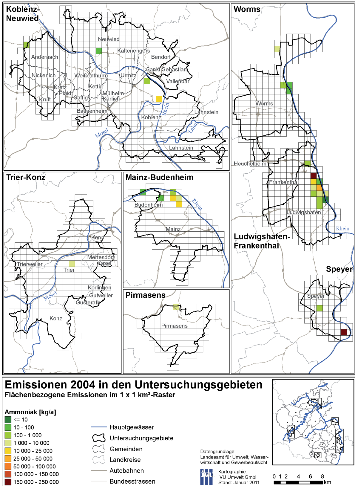
Abb. 59: Flächenbezogene Ammoniak-Emissionen in den Untersuchungsgebieten 2004 im 1 x 1 km 2 -Raster
