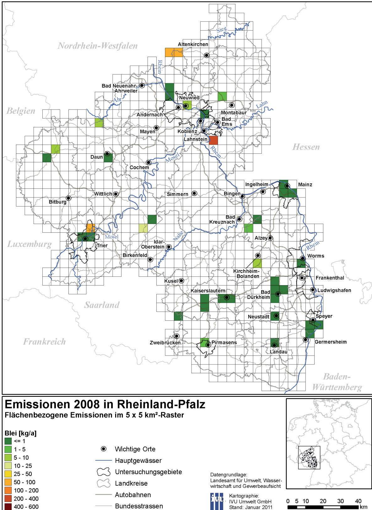
Abb. 56: Flächenbezogene Blei-Emissionen 2008 im 5 x 5 km 2 -Raster
