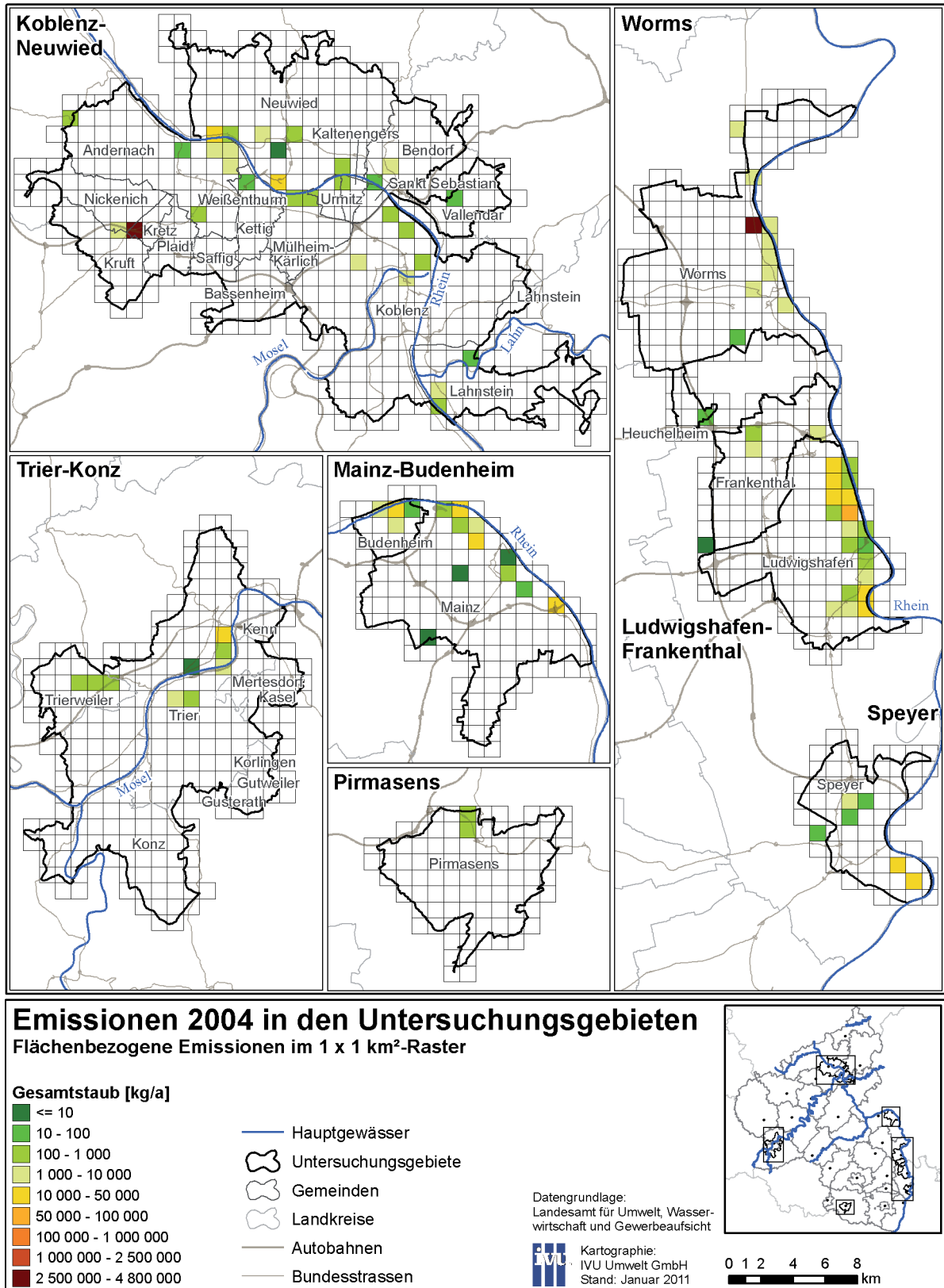
Abb. 79: Flächenbezogene Gesamtstaub-Emissionen in den Untersuchungsgebieten 2004 im 1 x 1 km 2 -Raster
