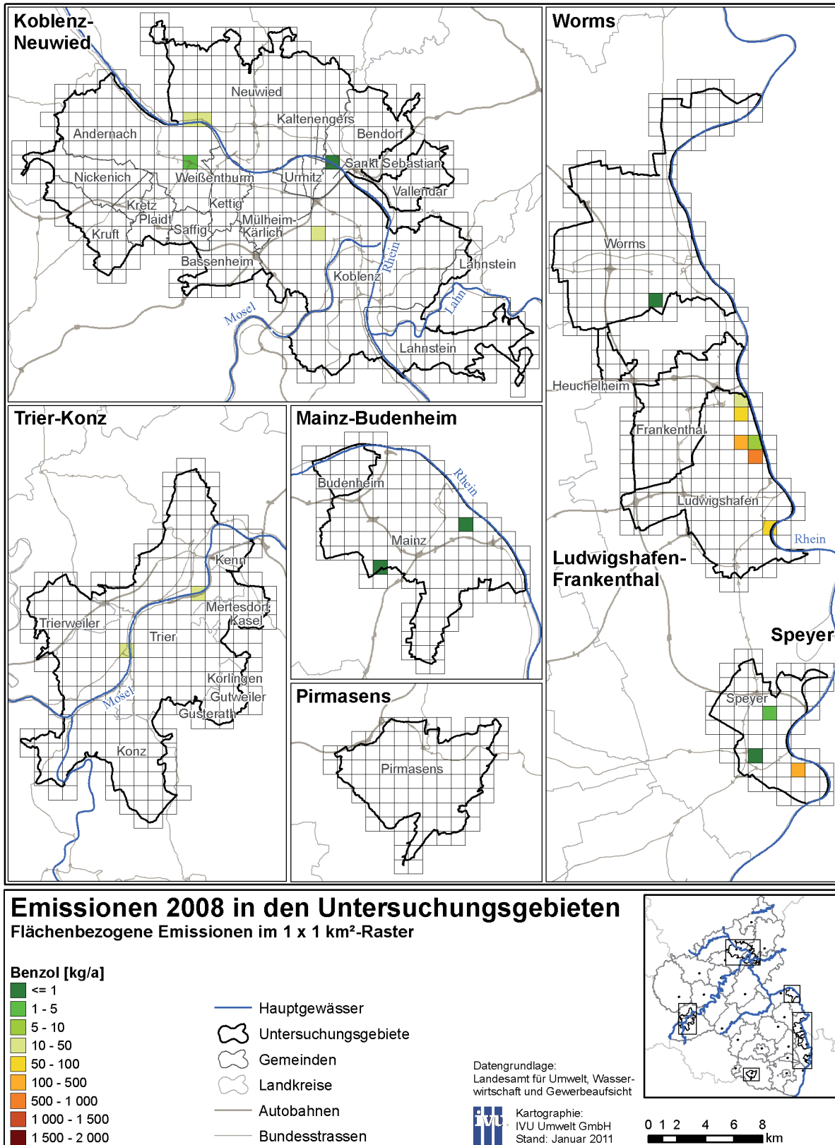
Abb. 74: Flächenbezogene Benzol-Emissionen in den Untersuchungsgebieten 2008 im 1 x 1 km 2 -Raster
