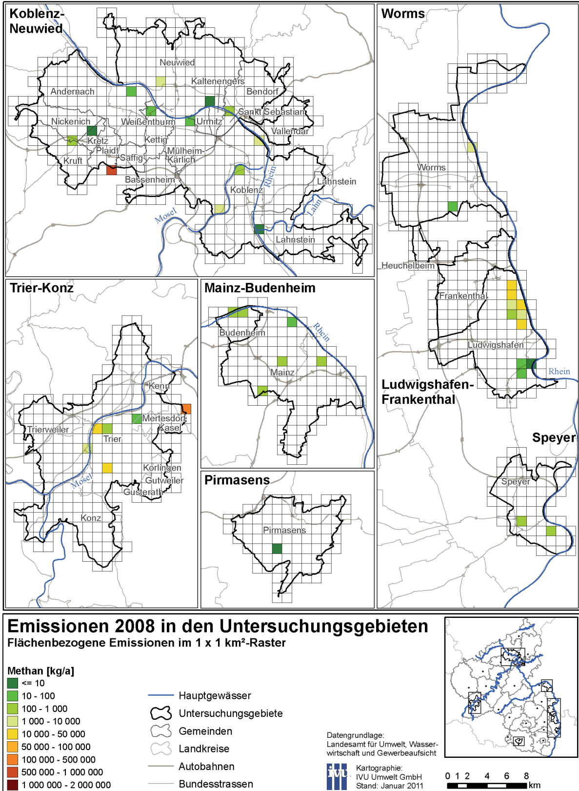
Abb. 76: Flächenbezogene Methan-Emissionen in den Untersuchungsgebieten 2008 im 1 x 1 km 2 -Raster
