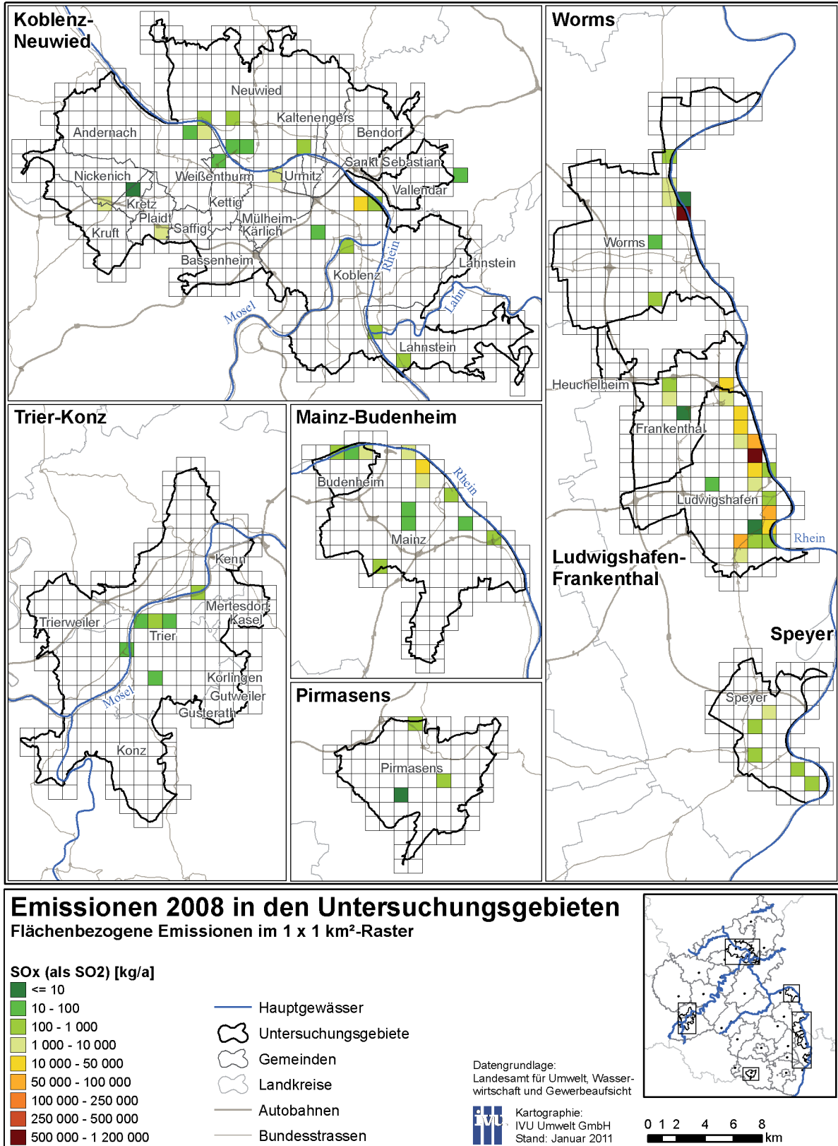
Abb. 70: Flächenbezogene Schwefeloxide-Emissionen in den Untersuchungsgebieten 2008 im 1 x 1 km 2 -Raster
