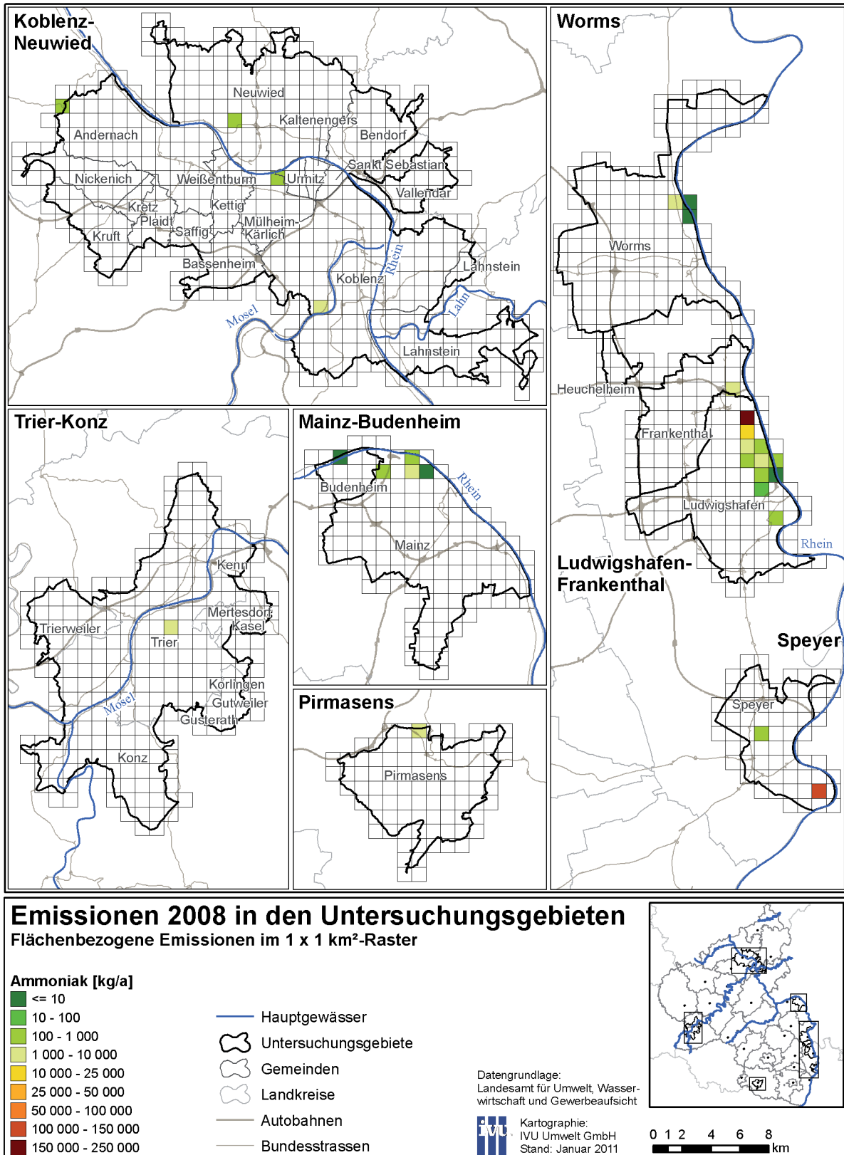
Abb. 60: Flächenbezogene Ammoniak-Emissionen in den Untersuchungsgebieten 2008 im 1 x 1 km 2 -Raster
