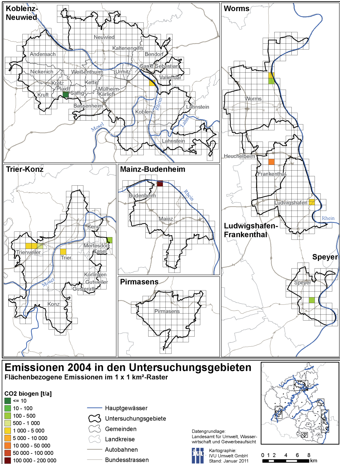
Abb. 65: Flächenbezogene biogene CO 2 -Emissionen in den Untersuchungsgebieten 2004 im 1 x 1 km 2 -Raster
