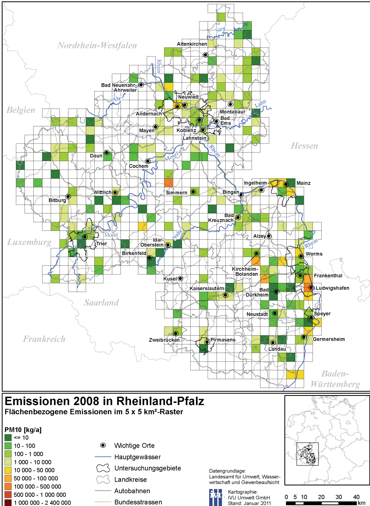
Abb. 52: Flächenbezogene PM10-Emissionen 2008 im 5 x 5 km 2 -Raster
