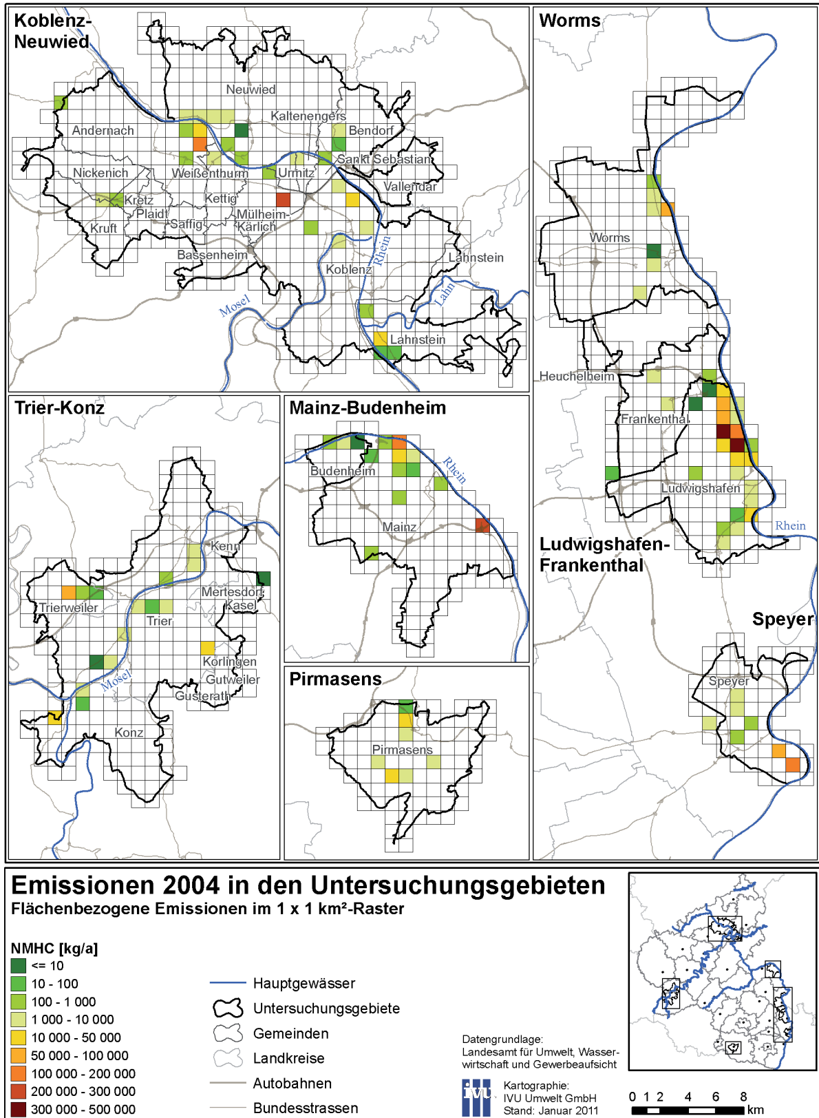
Abb. 77: Flächenbezogene NMHC-Emissionen in den Untersuchungsgebieten 2004 im 1 x 1 km 2 -Raster
