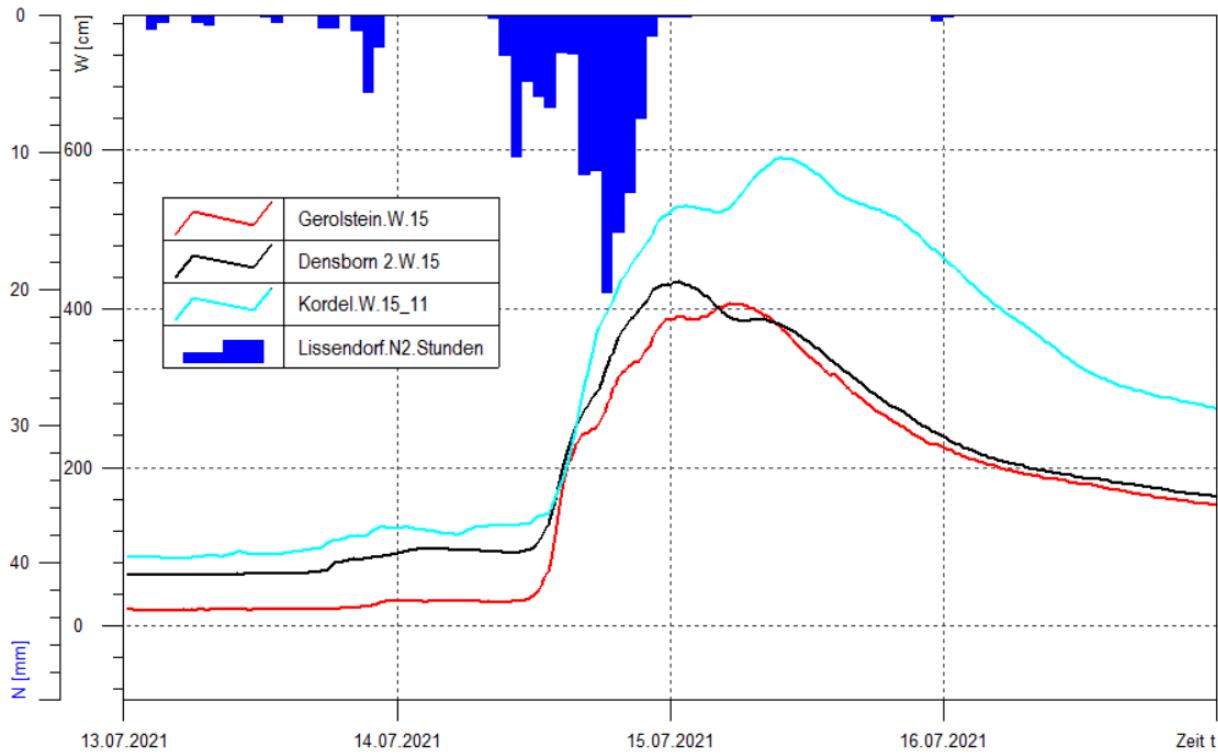
Abbildung 9: Niederschlag an der Messstation Lissendorf und Abflussreaktion an drei Pegeln an der Kyll.
