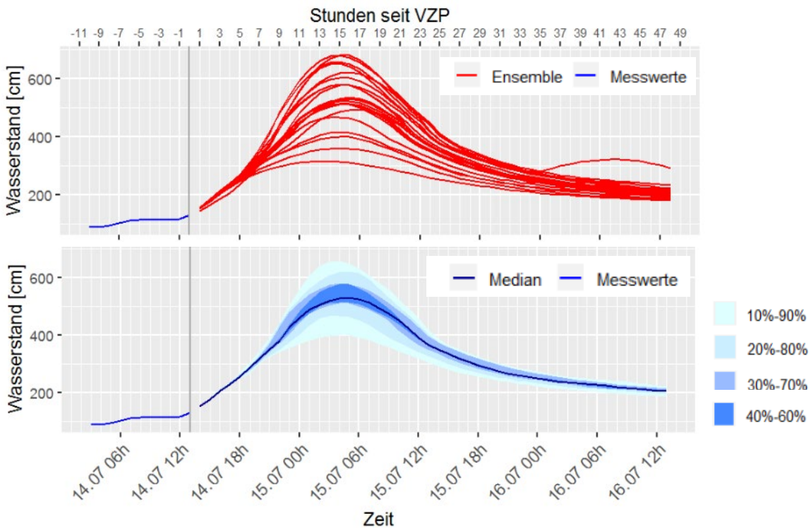
Abbildung 14: Spanne der Wasserstandsvorhersagen für den Pegel Altenahr zum Vorhersagezeitpunkt 14.07. 14:00 MESZ unter Verwendung von 20 Ensemble-Wettervorhersagen (ICON-D2-EPS); 20 Einzelvorhersagen (oben) und Quantildarstellung (unten).
