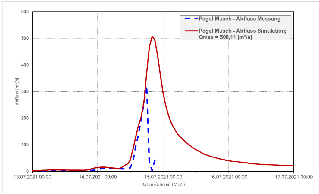
Abbildung 26: Gemessene (Daten 14.07. Uhr 19:30 – 22:00 Uhr unplausibel) und simulierte Abflussganglinie am Pegel Müsch
