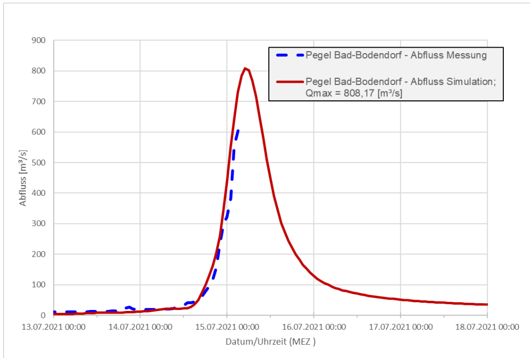
Abbildung 28: Gemessene und simulierte Abflussganglinie am Pegel Bad Bodendorf
