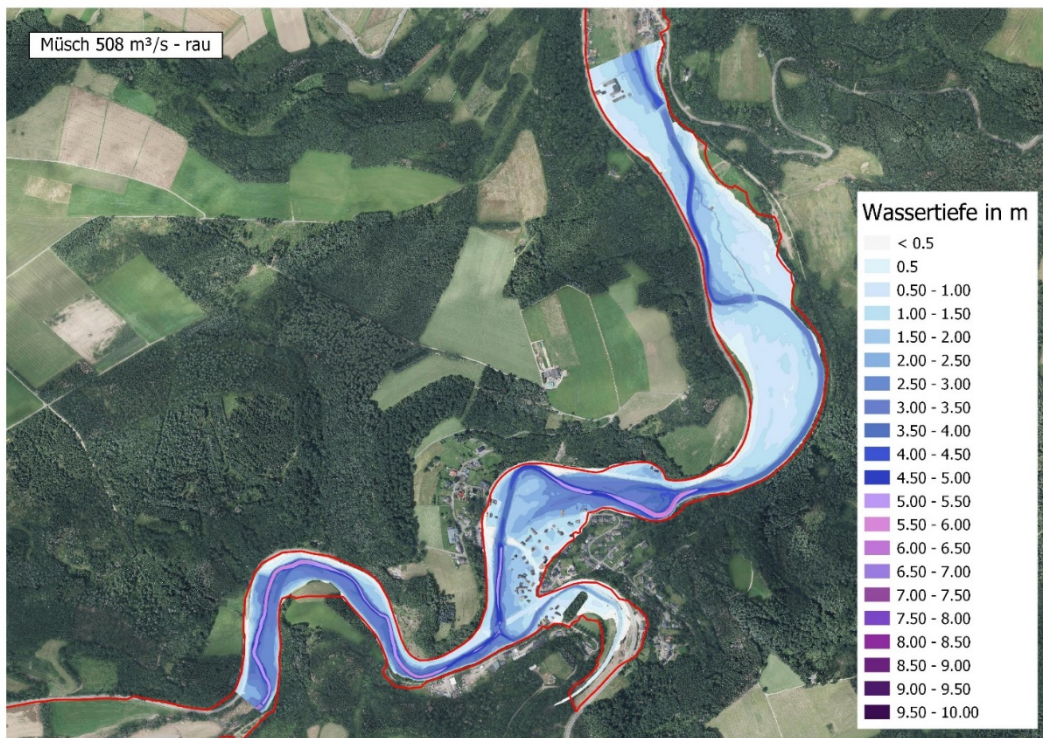
Abbildung 46: Rekonstruierte und berechnete Überschwemmungsflächen ( Q = 508 \text{ m}^3/\text{s} , unverklast) im Bereich des Pegels Müsch (Vorland und Flussschlauch rauer) (Datengrundlage: Geobasisinformationen der Vermessungs- und Katasterverwaltung).
