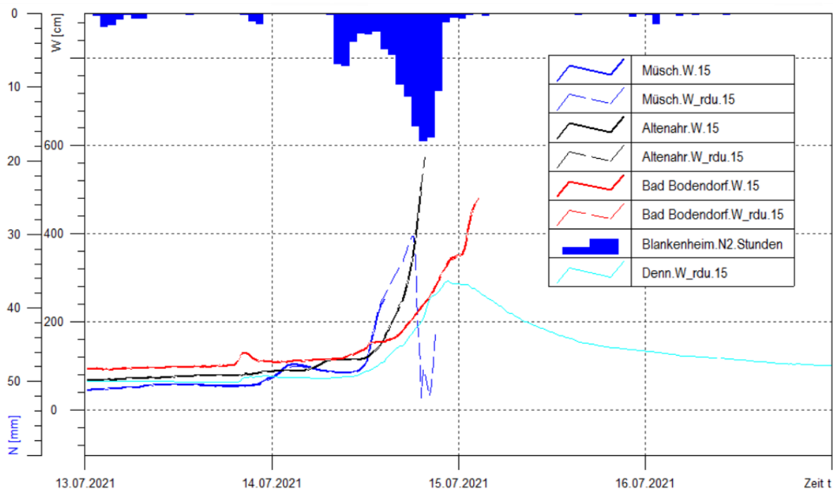
Abbildung 8: Niederschlag an der Messstation Blankenheim und Abflussreaktion an vier Pegeln im Ahr-Einzugsgebiet; für Müsch, Altenahr und Bad Bodendorf jeweils Darstellung von Hauptgeber (W.15) und redundantem Messsensor (W_rdu.15).
