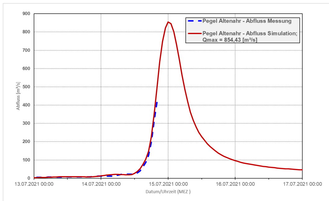
Abbildung 27: Gemessene und simulierte Abflussganglinie am Pegel Altenahr
