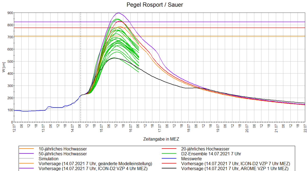
Abbildung 12: Wasserstandsvorhersagen am 14.07. mit VZP 07:00 Uhr und Darstellung des Vorhersageensembles am Pegel Rosport (lila: mit ICON-D2 VZP 04:00, rot: mit ICON-D2 VZP 07:00, orange: geänderte Modelleinstellung, schwarz: AROME VZP 01:00, grün: Ensemble VZP 07:00); alle Zeitangaben in MEZ.
