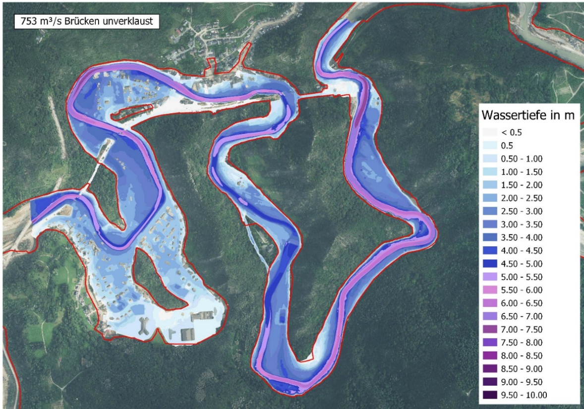
Abbildung 42: Rekonstruierte und berechnete ( Q = 753 \text{ m}^3/\text{s} , unverklast) Überschwemmungsflächen im Bereich des Pegels Altenahr (Datengrundlage: Geobasisinformationen der Vermessungs- und Katasterverwaltung).
