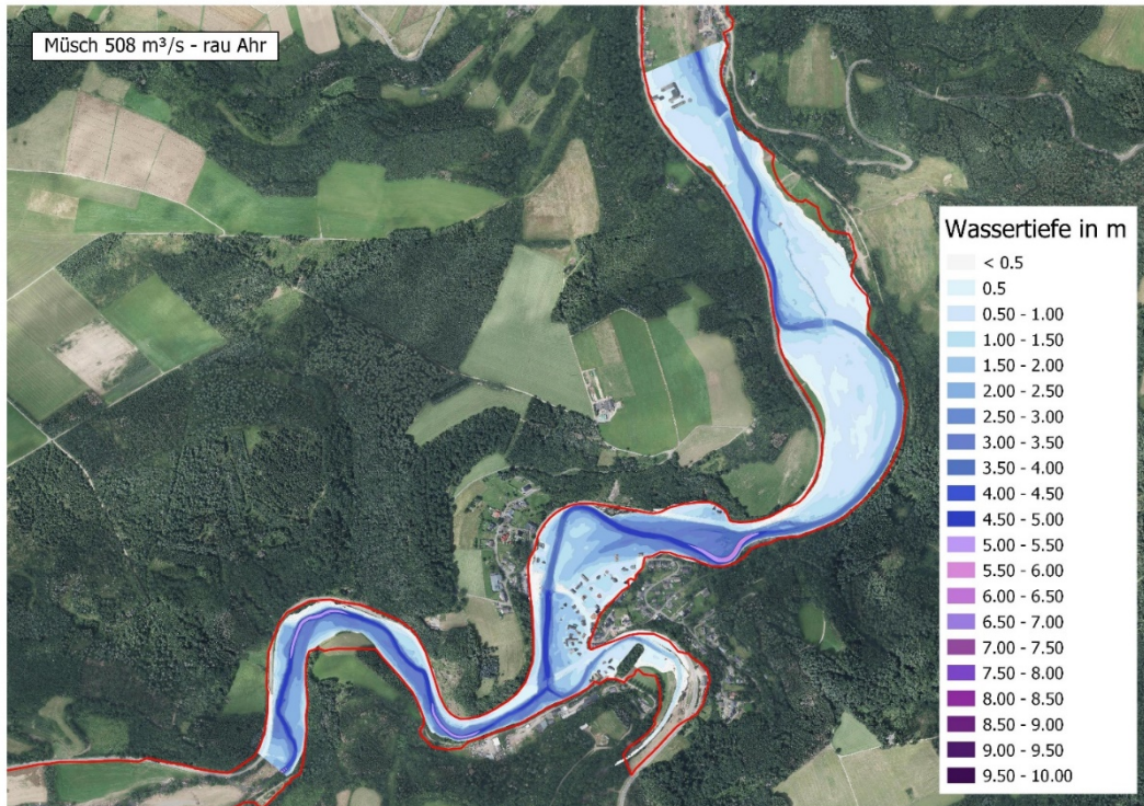
Abbildung 47: Rekonstruierte und berechnete Überschwemmungsflächen ( Q = 508 \text{ m}^3/\text{s} , unverklast) im Bereich des Pegels Müsch (Flussschlauch rau) (Datengrundlage: Geobasisinformationen der Vermessungs- und Katasterverwaltung).
