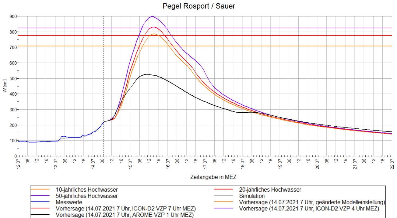
Abbildung 11: Wasserstandsvorhersagen am 14.07. mit VZP 07:00 Uhr am Pegel Rosport (lila: mit ICON-D2 VZP 04:00, rot: mit ICON-D2 VZP 07:00, orange: geänderte Modelleinstellung, schwarz: AROME VZP 01:00), alle Zeitangaben in MEZ.
