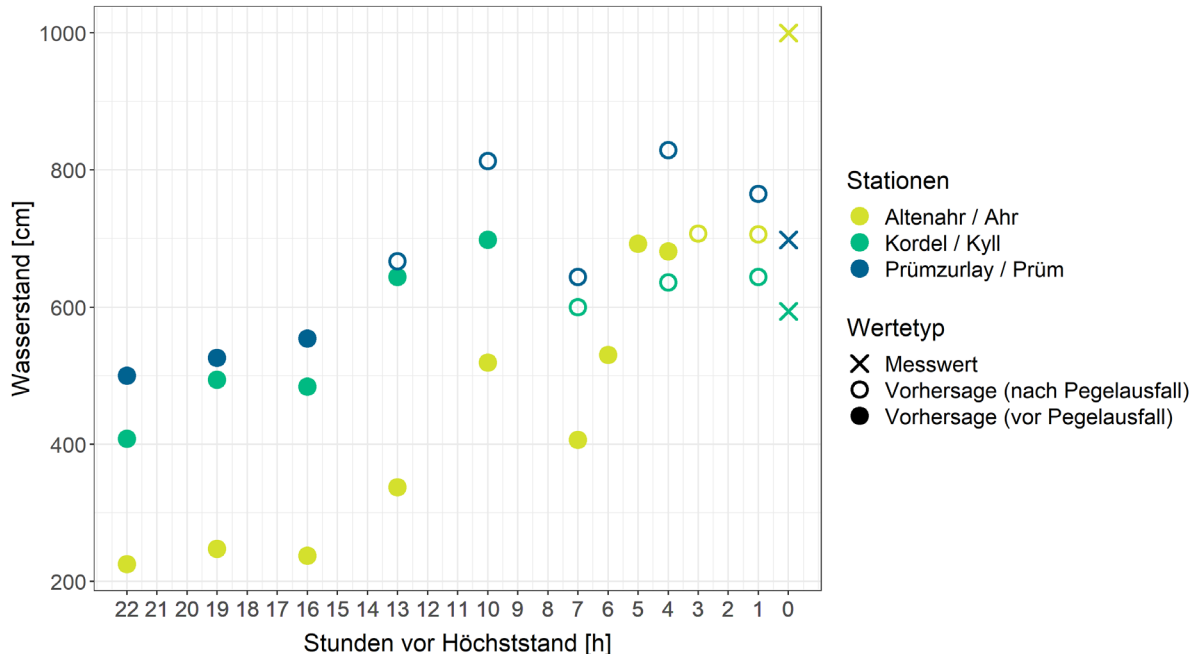
Abbildung 13: Vorhergesagte Höchststände für die Pegel Altenahr, Kordel und Prümzurley für Vorhersagezeitpunkte vor dem gemessenen Höchststand („gemessener“ Höchststand für Altenahr rekonstruiert).
