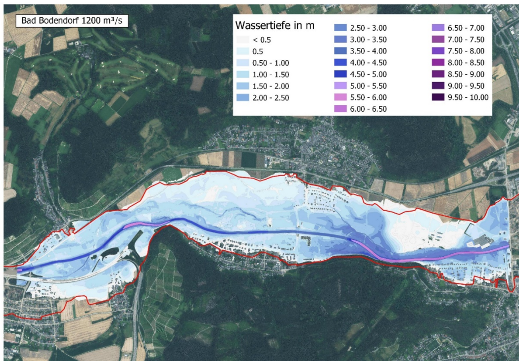
Abbildung 35: Rekonstruierte (Anschlagslinie) und berechnete ( Q = 1.200 \text{ m}^3/\text{s} ) Überschwemmungsflächen im Bereich des Pegels Bad Bodendorf (Datengrundlage: Geobasisinformationen der Vermessungs- und Katasterverwaltung).
