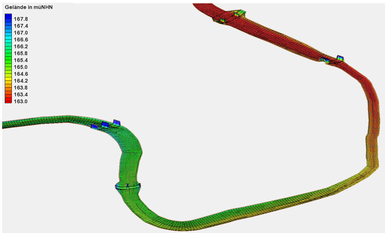
Abbildung 29: Ausschnitt aus dem 3D-Flussschlauch der Ahr im Bereich des Pegelmodells Altenahr mit eingearbeiteten Brückenwiderlagern und -pfeilern (Datengrundlage: Geobasisinformationen der Vermessungs- und Katasterverwaltung).
