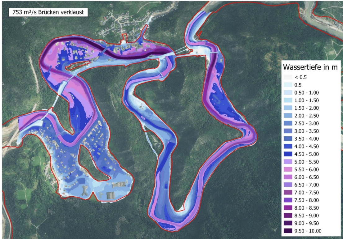
Abbildung 43: Rekonstruierte und berechnete ( Q = 753 \text{ m}^3/\text{s} , verklaut) Überschwemmungsflächen im Bereich des Pegels Altenahr (Datengrundlage: Geobasisinformationen der Vermessungs- und Katasterverwaltung).
