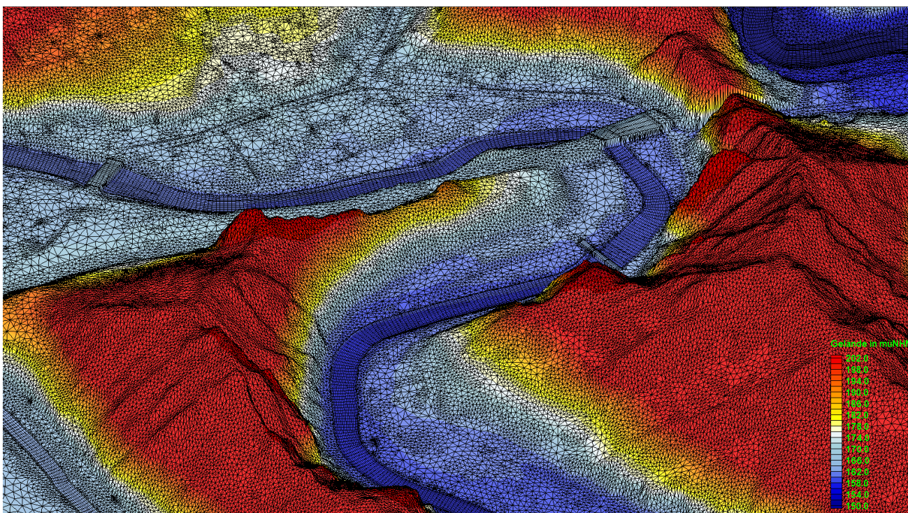
Abbildung 31: Ausschnitt aus dem Pegelmodell Altenahr, Nachbildung der Brücken als vollständig verlegt (Datengrundlage: Geobasisinformationen der Vermessungs- und Katasterverwaltung).
