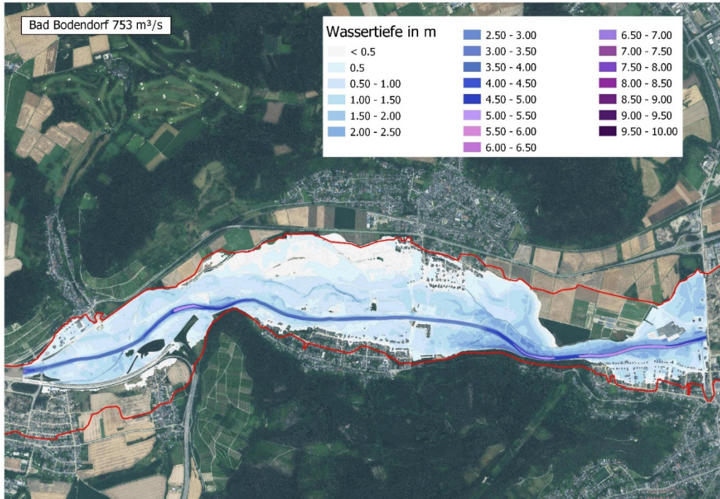
Abbildung 34: Rekonstruierte (Anschlagslinie) und berechnete ( Q = 753 \text{ m}^3/\text{s} ) Überschwemmungsflächen im Bereich des Pegels Bad Bodendorf (Datengrundlage: Geobasisinformationen der Vermessungs- und Katasterverwaltung).
