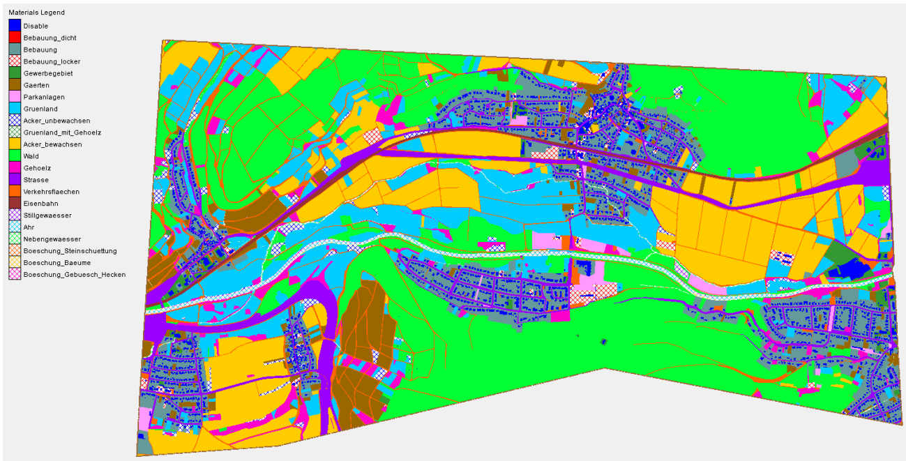
Abbildung 30: Materialbelegung im Pegelmodell Bad Bodendorf (Datengrundlage: Geobasisinformationen der Vermessungs- und Katasterverwaltung).
