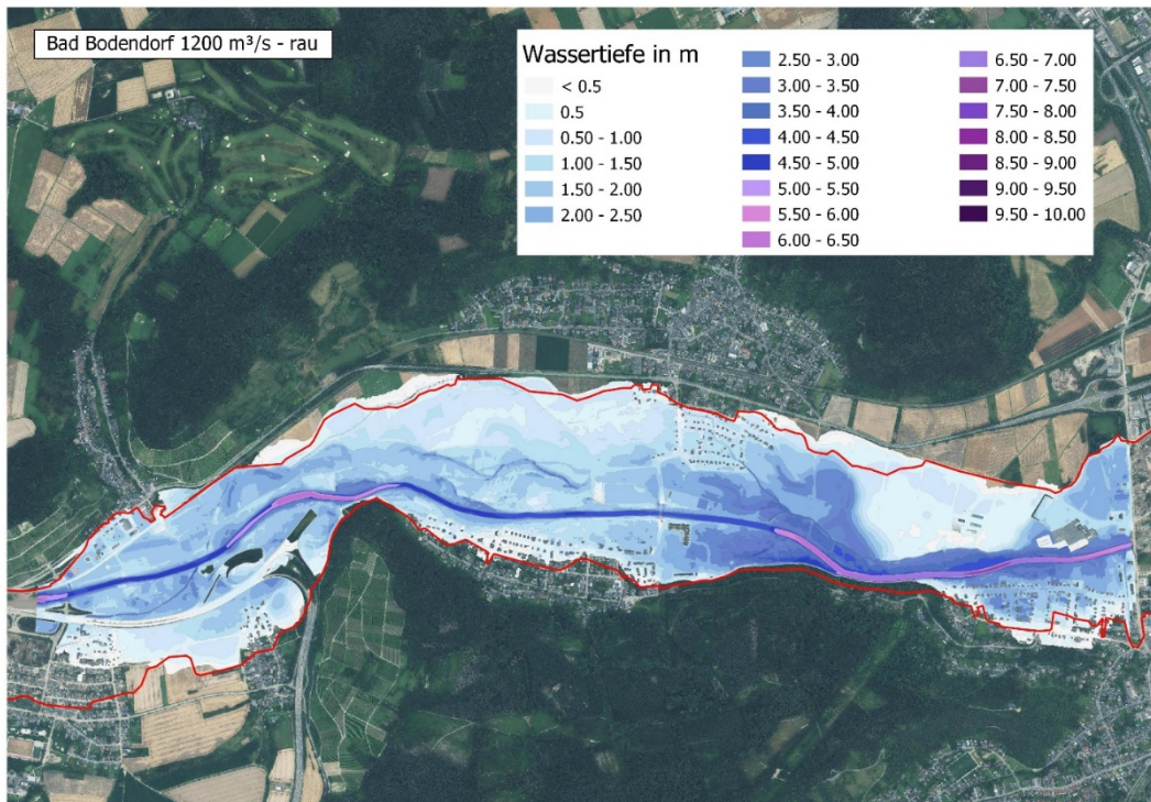
Abbildung 36: Rekonstruierte (Anschlaglinie) und berechnete ( Q = 1.200 \text{ m}^3/\text{s} , raue Variante) Überschwemmungsflächen im Bereich des Pegels Bad Bodendorf (Datengrundlage: Geobasisinformationen der Vermessungs- und Katasterverwaltung).
